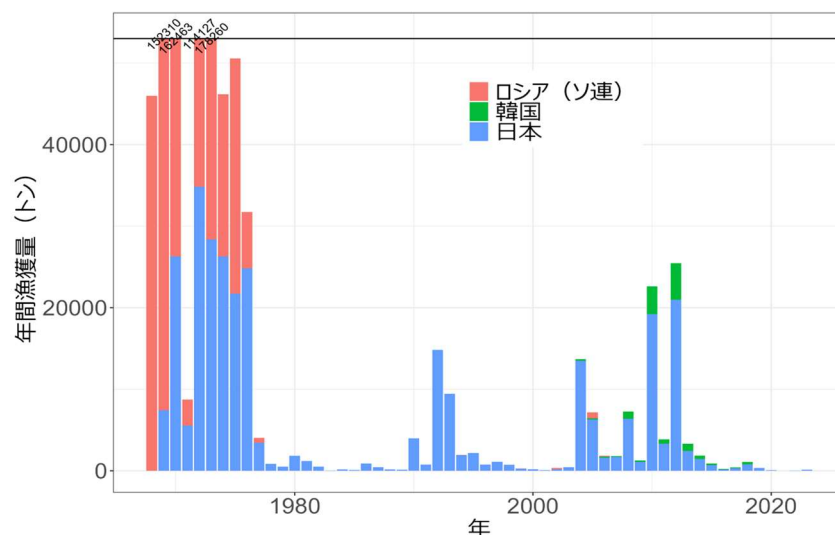
図 2. 天皇海山海域におけるクサカリツボダイ国別漁獲量の推移 (1968～2023 年)
