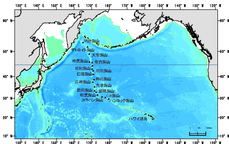
図 1. 天皇海山海域の主要海山群
