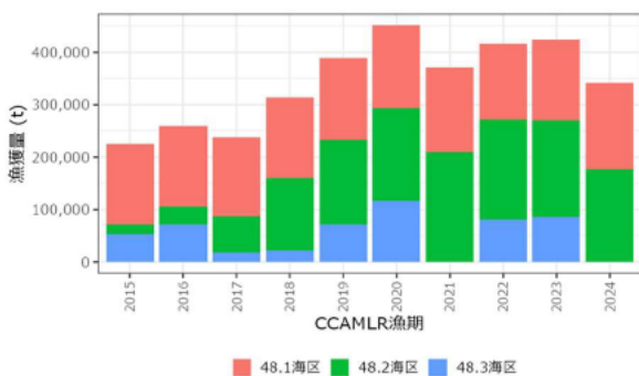
48海区における過去10年間の小海区分別 ナンキョクオキアミ漁獲量 (2014/15~2023/24漁期) 2023/24漁期の漁獲量は2024年5月31日時点。
