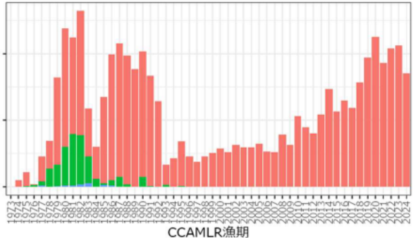
ナンキョクオキアミの海区別漁獲量の経年変化 (1972/73~2023/24 漁期) 2023/24 漁期の漁獲量は2024年5月31日時点。
