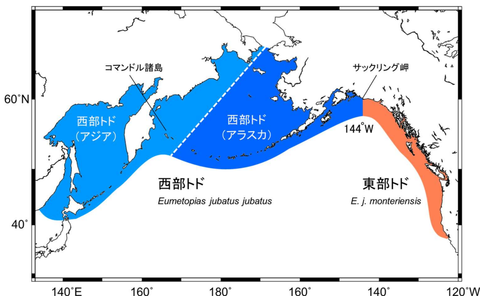
図3. トドの分布 (Loughlin 1997 及び Young et al. 2024 に基づく)
