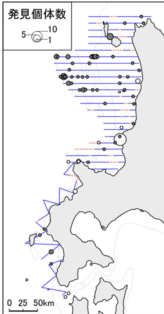
図8. 航空機目視調査の調査定線とトド発見位置 (2013年、Hattori et al. 2021に基づく)
