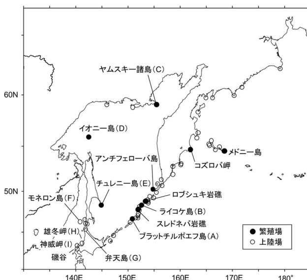
図4. 西部トド (アジア) の繁殖場及び上陸場の分布 (Burkanov and Loughlin 2005 に基づく)
