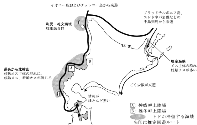
図9. 1980年代の回遊模式図(山中ほか1986)
