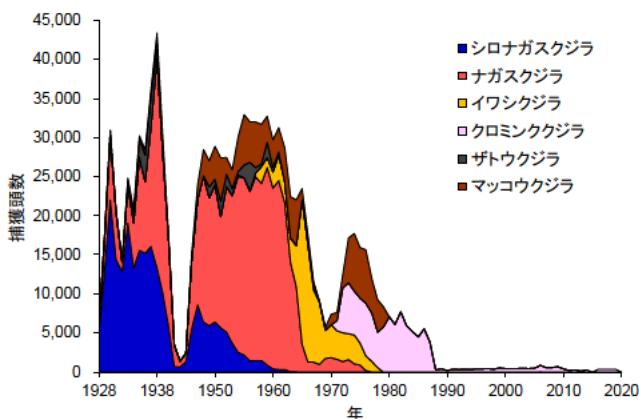
図 1. 1928 年から 1986/87 年までの南極海母船式捕鯨によるシロナガスクジラ (濃青色) 捕獲頭数の変遷、1987/88 年以降は調査による標本採集数の変遷 データ出典：Allison 2016、水産庁ウェブページ (「捕鯨の部屋 鯨類科学調査」)。
