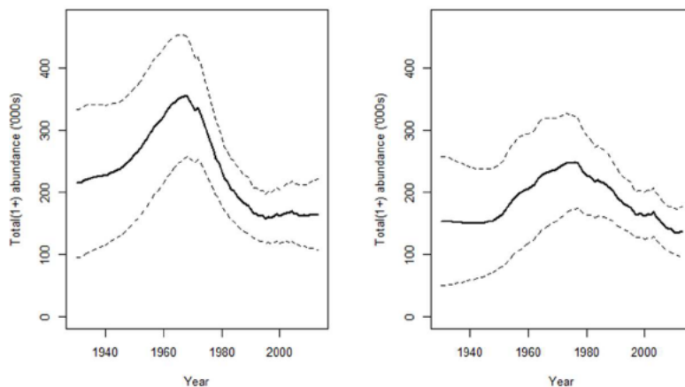
SCAA により推定したクロミンクジラのインド洋系群 (左) 及び太平洋系群 (右) の 1 歳以上の資源量 (頭数)
