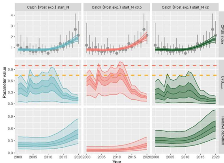
図 6. 南西太平洋のクロトガリザメの標準化 CPUE の年トレンド（上段）、長期的に資源が絶滅する水準の漁獲死亡係数（ U_{\text{crash}} ）に対する各年の漁獲死亡係数（中段）、及び漁業による開発前の資源量に対する各年の資源量の変化（下段）（WCPFC 2024）。
