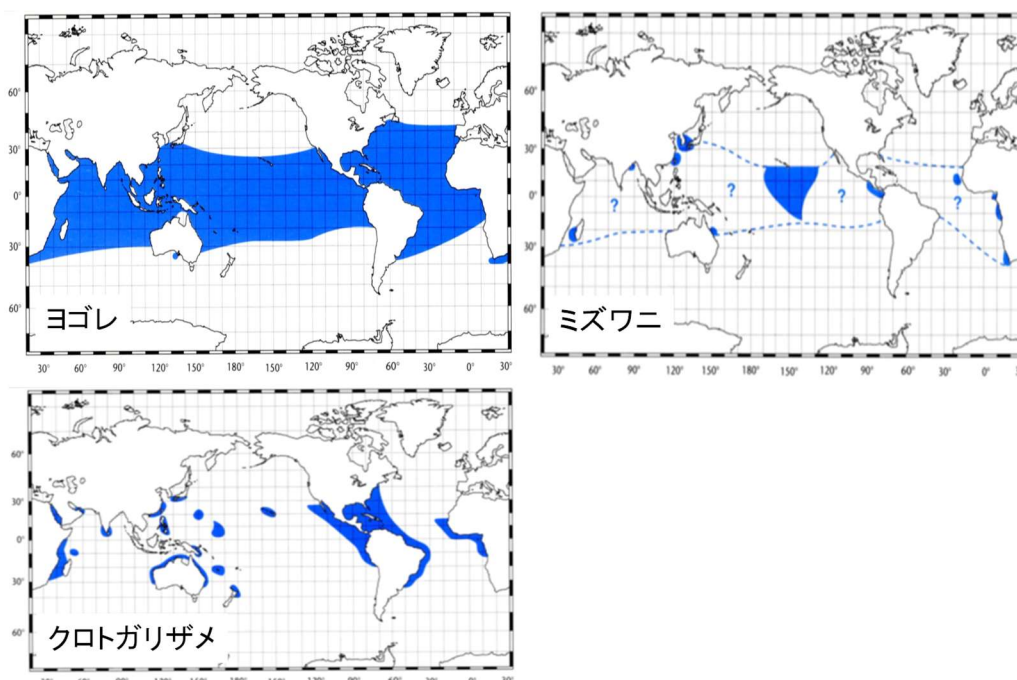
図 1. 外洋性サメ類の分布（Last and Stevens 1994）
