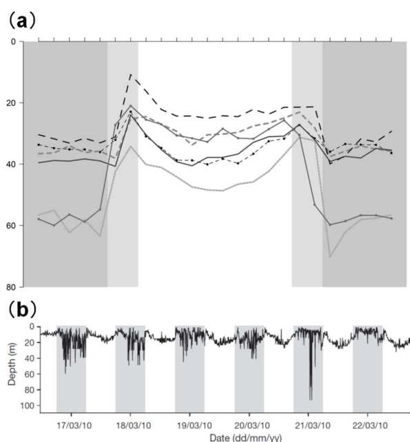
図 2. FAD に網集する (a) ヨゴレと (b) クロトガリザメの日周鉛直移動
