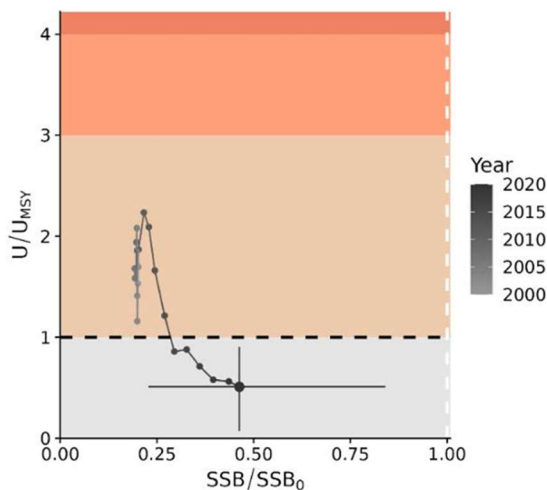
図 7. 南西太平洋のクロトガリザメの資源状態の年変化 (WCPFC 2024)。
