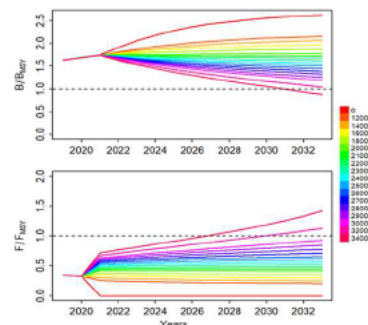
JABBAによる将来予測(2021～2033年)。上図は相対的資源量 ( B/B_{MSY} ) と下図は相対的漁獲係数 ( F/F_{MSY} )。色線は漁獲量を0～34,000トンまで変化した際のそれぞれの将来予測軌道。各線は15,000回のマルコフ連鎖モンテカルロ法によるシミュレーション結果の中央値。
