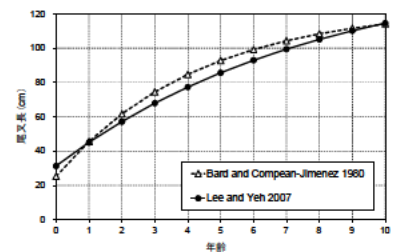
南大西洋におけるビンナガの成長曲線
