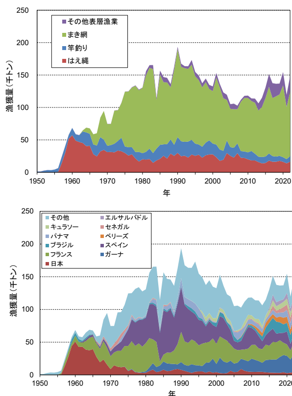
図1. 大西洋におけるキハダの漁法別漁獲量(1950~2022年、上図)と国・地域別漁獲量(1950年~2022年、下図)
