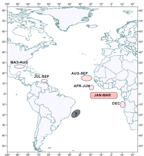
図 4. 大西洋におけるキハダの産卵場と産卵期 (月)
