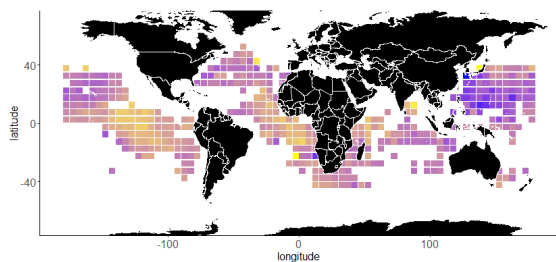
図 5. 各大洋における日本はえ縄漁業によるキハダの平均漁獲物サイズ (尾叉長 cm) の一例 (2000 年代)
