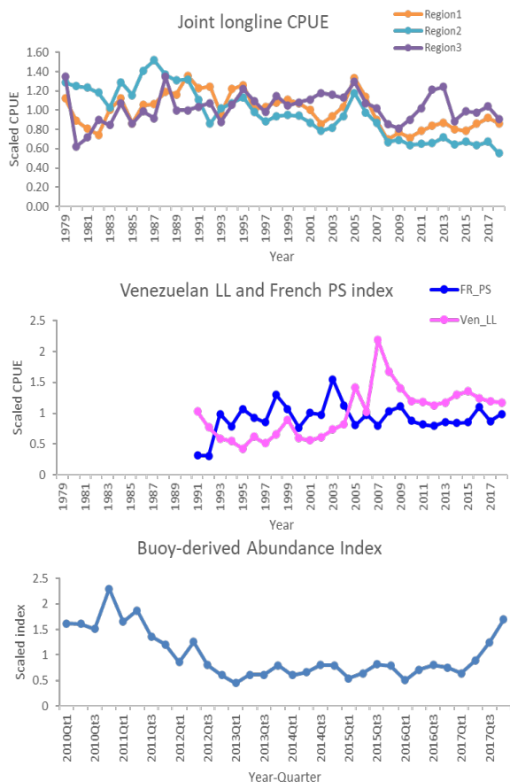
図7. 大西洋におけるキハダの資源量指数
