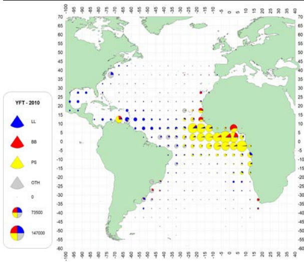
図 2. 大西洋におけるキハダの漁場（漁獲分布、2010～2019 年）
