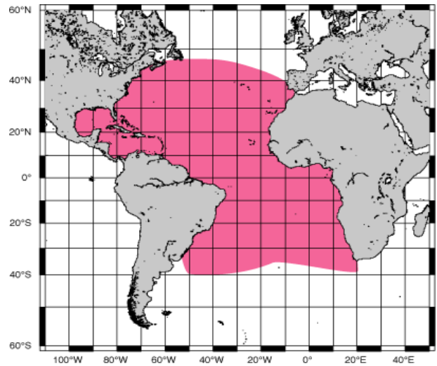
図 3. 大西洋におけるキハダの分布域
