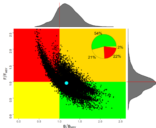
図9. 大西洋キハダの資源解析結果（各モデルの結果を統合）
