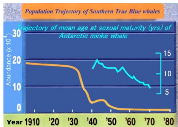
図3. 通常型シロナガスクジラの資源量減少（オレンジ色）とクロミンククジラの早熟化（青色）（加藤 1998）
