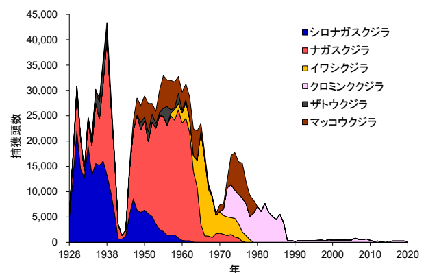
ナガスクジラ(濃青色)捕獲頭数の変遷、1987/88年以降は調査による標本採集数の変遷
