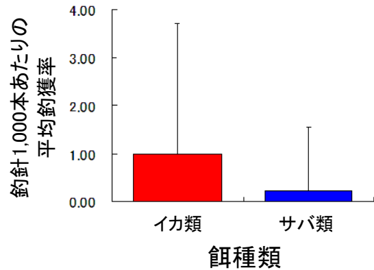
図5. イカ餌とサバ餌によるアカウミガメの混獲率 (Yokota et al. 2009の図を改変)
