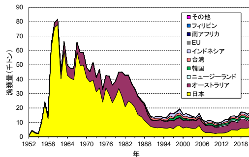
ミナミマグロの国・地域別漁獲量の推移 (1952～2021年)
