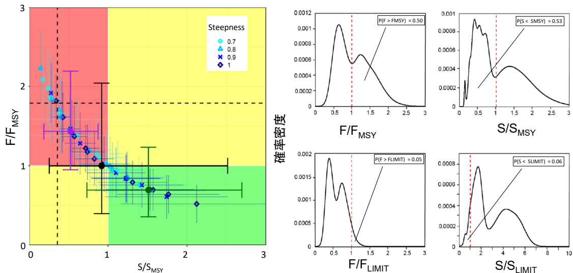
図5. 東部太平洋における最新年のメバチの資源状態（左）及び暫定目標管理基準値（MSY）と暫定限界管理基準値（LIMIT）を超える割合（中：漁獲の強さ。右：資源量）
