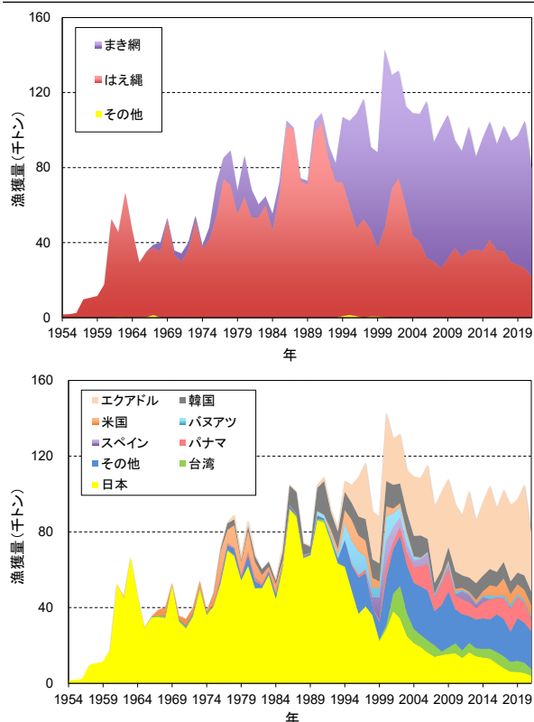
図 2. 東部太平洋におけるメバチの漁法別漁獲量（上図）、国・地域別漁獲量（下図）（1954～2021 年）
