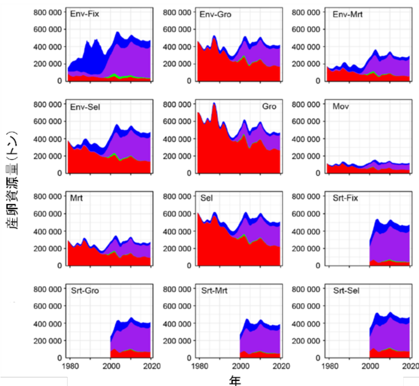
図 9. 東部太平洋におけるメバチの産卵魚資源量と各漁業のインパクトの推移 (1979～2020 年)
