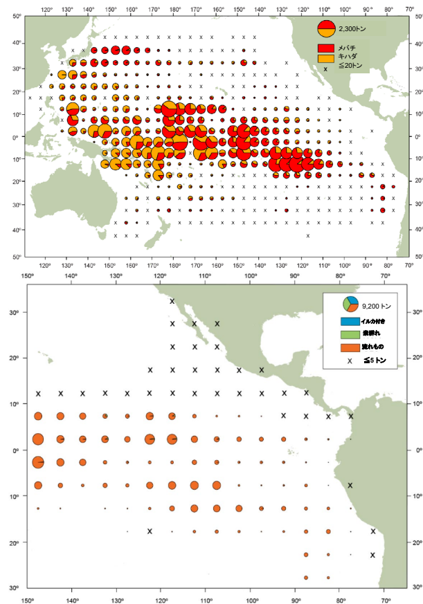
図 3. 太平洋における漁場図（上：はえ縄、下：ますき網）（上：2016～2020 年平均、下：2021 年）
