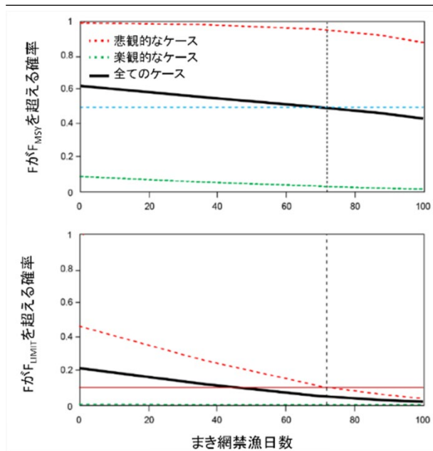
図 10. 東部太平洋におけるメバチのまき網禁漁日数と暫定目標管理基準値、暫定限界管理基準値を超える確率の関係 赤破線：悲観的なケースの平均。緑破線：楽観的なケースの平均。黒実線：全てのケースの平均。まき網禁漁日数と漁獲死亡率が暫定管理基準値 ( F_{MSY} ; 上図)、暫定限界管理基準値を超える確率 ( F_{LIMIT} ; 下図)。垂直の点線は 2018～2020 年まで適用された 72 日間のまき網禁漁日数を示す。
