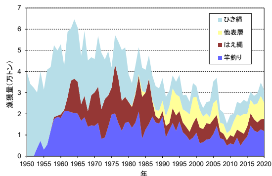
北大西洋におけるビンナガの漁法別漁獲量 (1950~2020 年)
