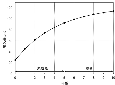
北大西洋ビンナガの成長曲線
