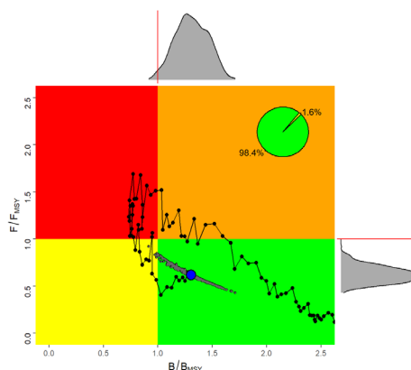
北大西洋ビンナガの資源における相対資源量 ( B/B_{MSY} ) と相対漁獲係数 ( F/F_{MSY} ) の推移 (1930~2018 年) 黒線: 資源状態の軌跡、黒点: 年別の資源状態、青点: 2018 年の資源状態、灰色点: 2018 年の資源状態の不確実性を示す。
