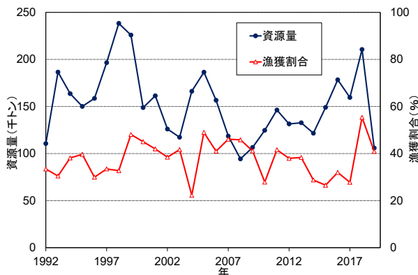
図 15. ゴマサバ東シナ海系群の資源量と漁獲割合(1992~2019年)
