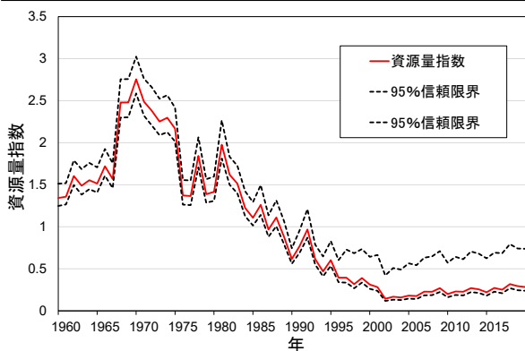
図7-1. 以底びき網(2そうびき)によるタチウオの資源量指数 (1959~2019年、MARSSモデル)
