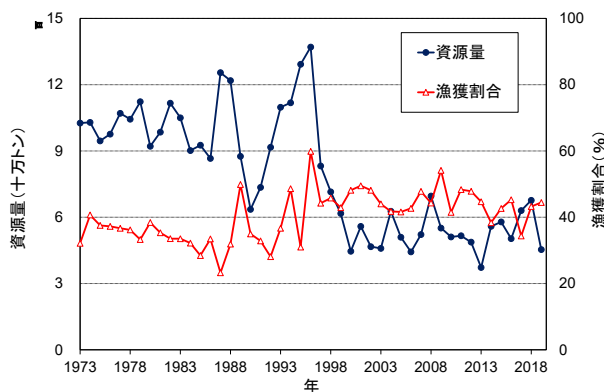
図11. マサバ対馬暖流系群の資源量と漁獲割合(1973~2019年)
