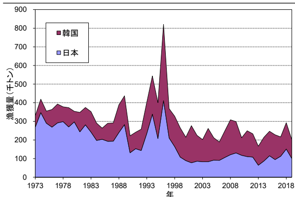
図9. マサバ対馬暖流系群の漁獲量(1973~2019年)
