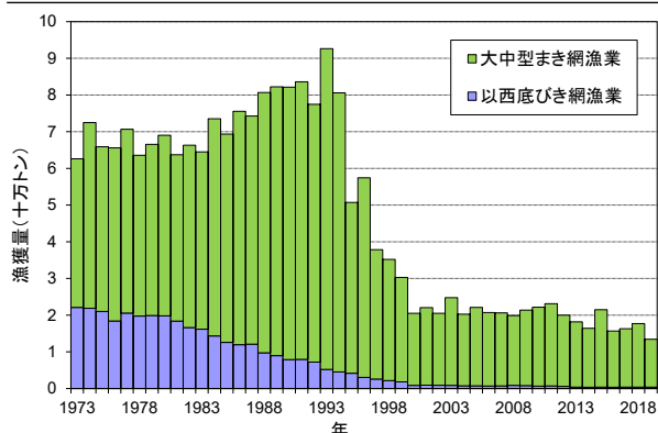
図 3. 以西底びき網漁業及び大中型まき網漁業の漁獲量の推移 (1973~2019年)
