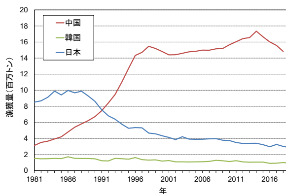
図2. FAO統計(北西太平洋区分)における日本、中国及び韓国の総漁獲量(1981~2019年)
