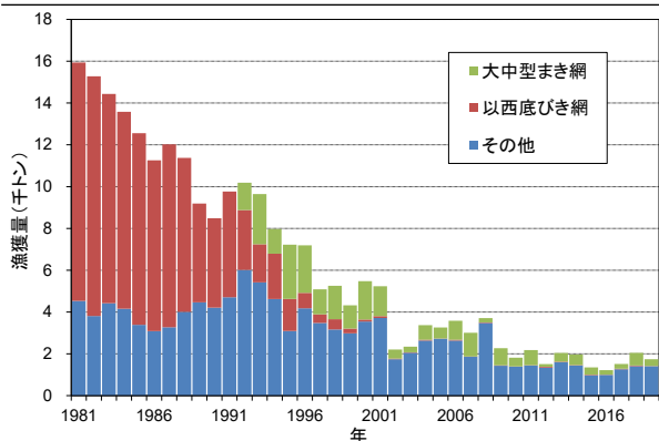
図 4-1. 我が国のタチウオ日本海・東シナ海系群の漁獲量 (1981～2019年)
