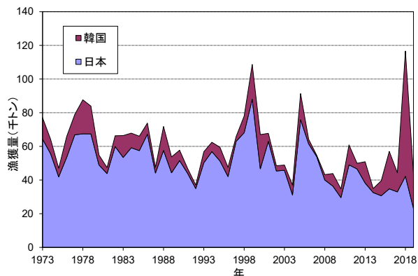
図 13. ゴマサバ東シナ海系群の漁獲量 (1973~2019年)
