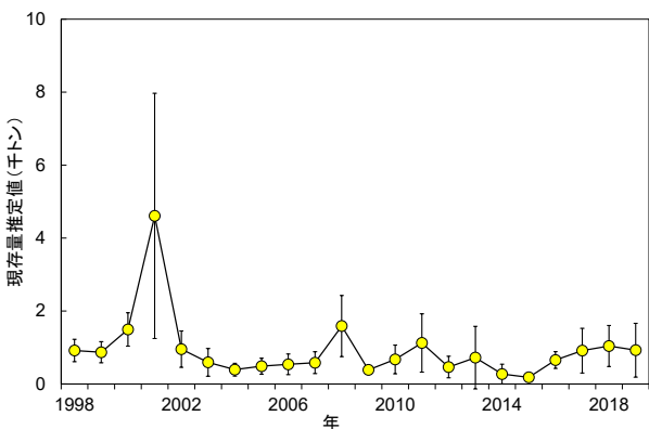
図7-2. 調査船トロール調査に基づく東シナ海タチウオの現存量推定値 (1998~2019年)
