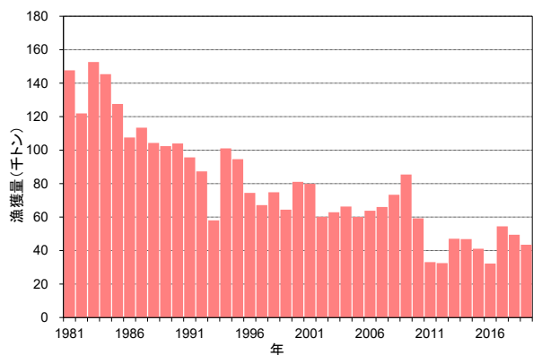
図 4-2. 韓国のタチウオ漁獲量 (1981～2019年)
