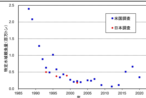
特定水域における日米調査船調査による中層性スケトウダラの現存量 (親魚量) 推定値
