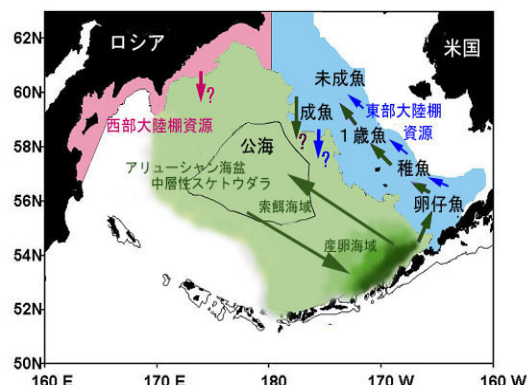
アリューシャン海盆の中層性スケトウダラの分布域 (緑) と想定される回遊経路略図
