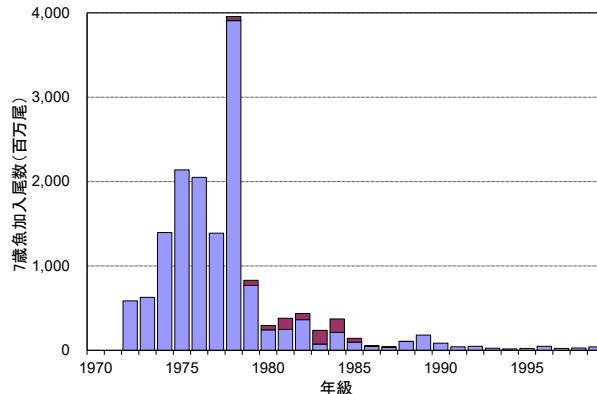
特定水域で米国調査により捕捉されたアリューシャン海盆への 7 歳魚加入尾数 1988 年以前の加入尾数は生残率から逆算された推定値を使用、赤は漁獲減耗。
