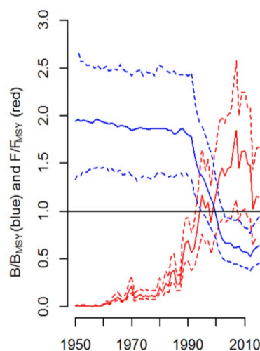
図5. BSP2で推定された相対資源量 ( B/B_{MSY} : 青線) 及び相対漁獲係数 ( F/F_{MSY} : 赤線) (ICCAT 2017)
