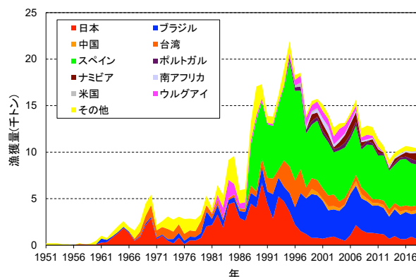
図2. 南大西洋におけるメカジキの国別漁獲量 (1951~2018年) (ICCAT 2020)
