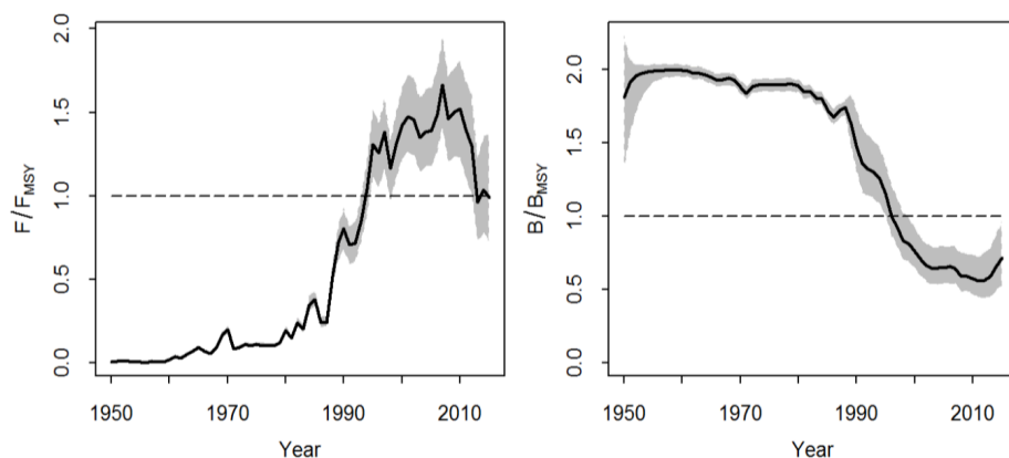
図 6. JABBA で推定された相対資源量 ( B/B_{MSY} : 右図) 及び相対漁獲係数 ( F/F_{MSY} : 左図) (ICCAT 2017) 灰色は 95%信頼区間。
