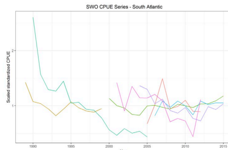
図4. 国別の標準化されたCPUE (ICCAT 2017)
