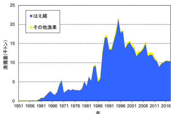
図1. 南大西洋におけるメカジキの漁法別漁獲量 (1951~2018年) (ICCAT 2020)
