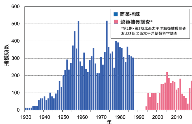
図 1. 北大西洋におけるミンククジラの捕鯨頭数の推移 (1930 ～ 2018 年) (定置網などによる混獲を含まない)
