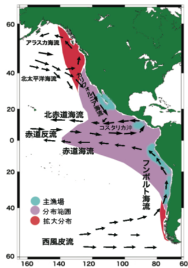
アメリカオオアカイカの分布と主な海流 ■の範囲はかつて報告されていた本種の分布範囲、■は最近年に分布拡大したと思われる範囲、■は主漁場。
