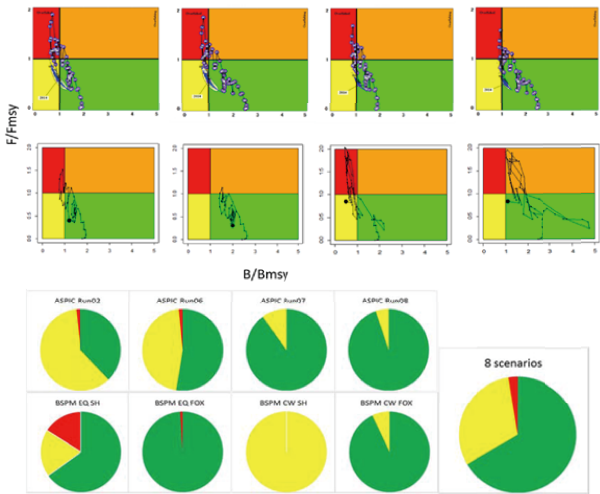
ASPIC モデル及び BSP モデルのそれぞれシナリオごとの Kobe plot (上段) と資源状態を確率として示した円グラフ (下段)
