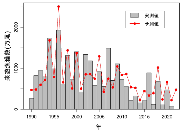
図 7. 日本系カラフトマスの来遊漁獲数の実測値と予測値の関係 (1990~2021 年)
