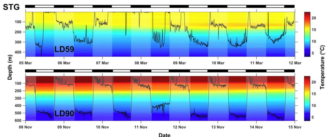
図 3-1. 北東太平洋において亜熱帯循環流を遊泳中のネズミザメ 2 個体の遊泳深度 (縦軸) と周辺水温の情報
