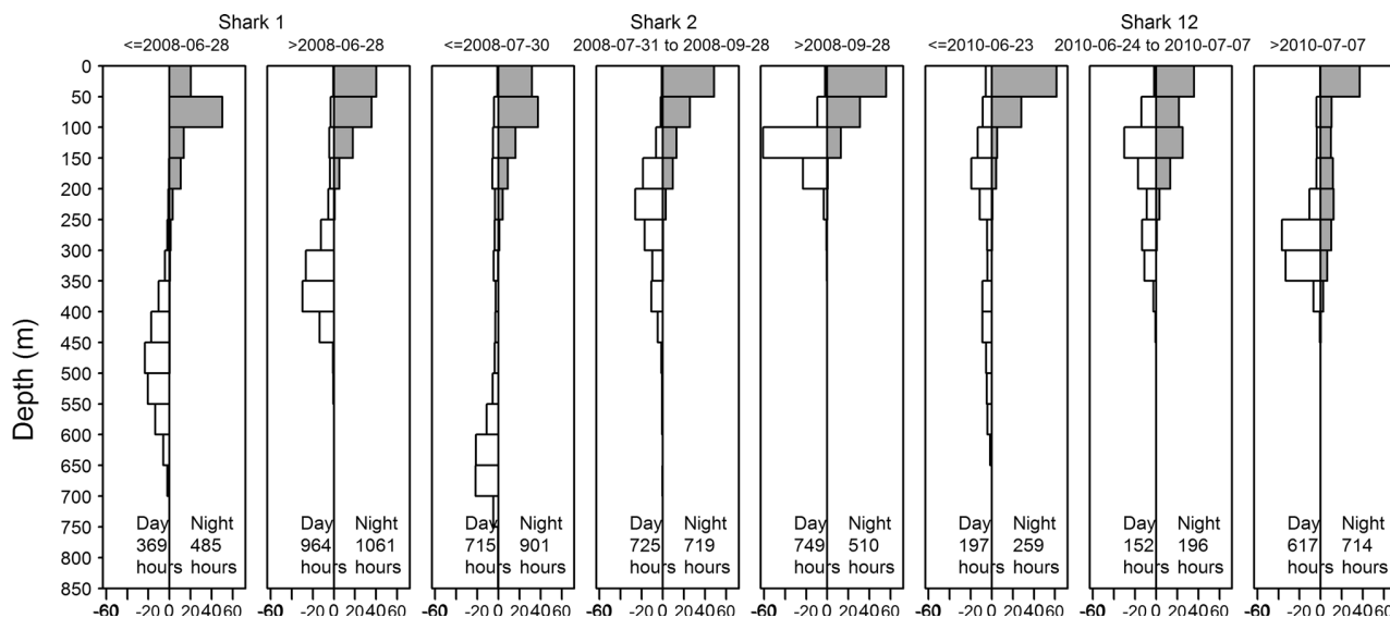
図 3-2. ニューゼaland近海で放流されたニシネズミザメ 3 個体 (Shark1、Shark2、Shark12) の昼夜別、水深帯別の滞在時間
