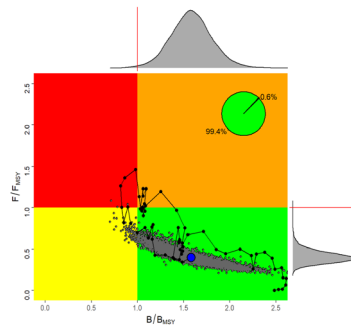
JABBAの神戸プロットと2018年の資源状態を確率として示した円グラフ
