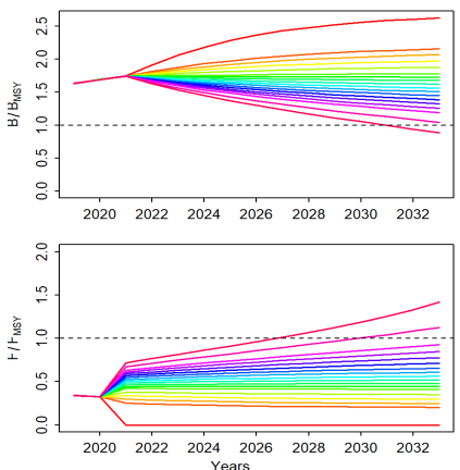
JABBAによる将来予測 (2021~2033年)
