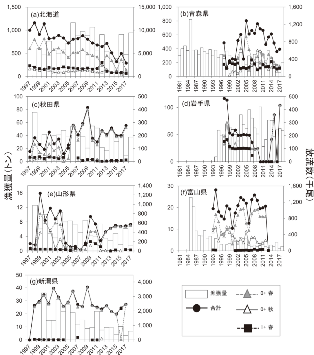
図4. 各道県におけるサクラマス漁獲量と放流数の推移
