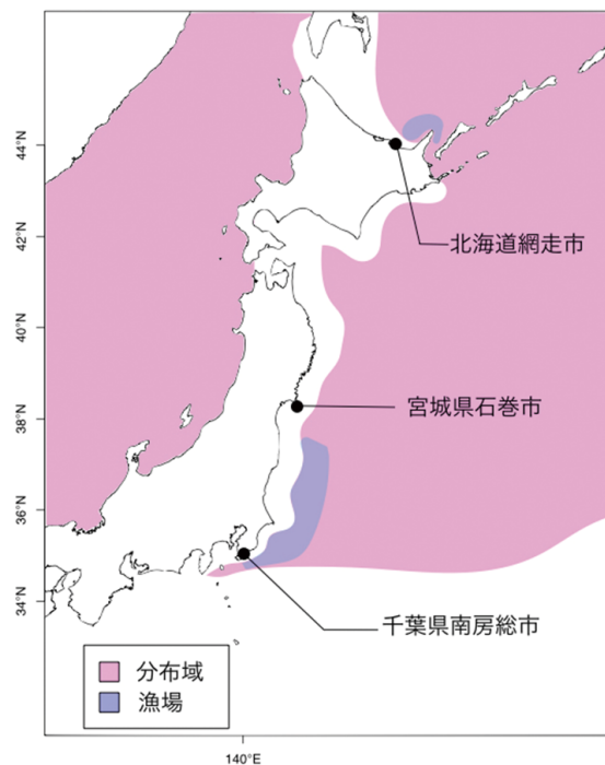
図3. 日本周辺におけるツチクジラの分布と漁場及び主な水揚地(鯨体処理場)
