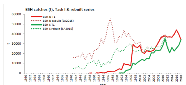
図4. 資源評価で用いられた北大西洋 (赤) と南大西洋 (緑) のヨシキリザメの推定漁獲量 (点線、1971～2012年) とICCATで集計している水揚げ量 (実線、1978-2018年) (ICCAT 2019)
