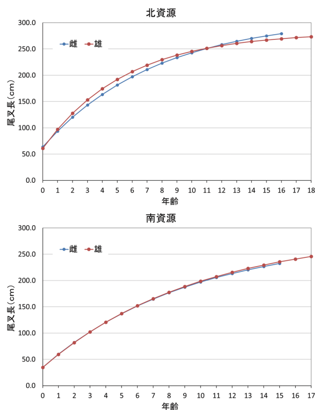
図3. ヨシキリザメの北資源 (Skomal and Natanson 2003) と南資源 (Mas 2015) の年齢と成長
