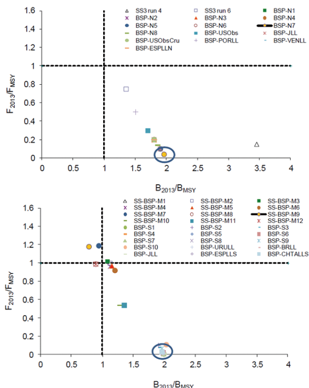
図6. 北資源に対して統合モデル(SS)及びベイジアンサープラスプロダクションモデル(BSP)で示された神戸プロット(上図)と、南資源に対してBSPと状態空間ベイジアンサープラスプロダクションモデル(SS-BSP)で示された神戸プロット(下図)(ICCAT 2019) 青いサークルはBSPで示された一般的な状態(2013年時点の資源状態は、乱獲状態ではなく過剰漁獲行為も行われていない状態)を表す。右上の凡例は、各モデルおよび複数の異なる設定で行われた感度解析を表す。例えば、SS3は統合モデルを表す。
