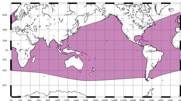
図2. ヨシキリザメの分布域 (Compagno 1984より)
