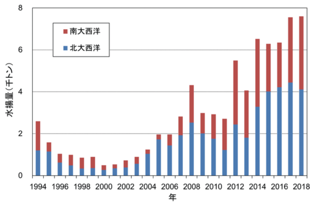
図1. 日本のヨシキリザメ(南北大西洋系群)の水揚げ量(1994～2018年)(データ:ICCAT 2019)
