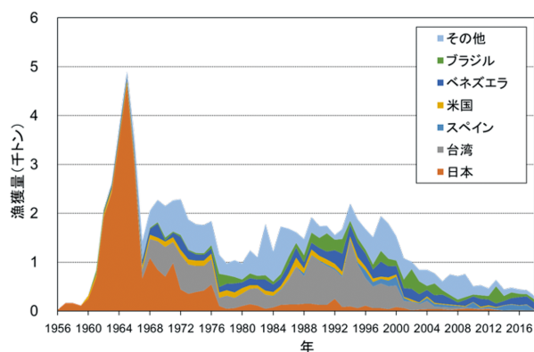
図1. ニシマカジキの国別漁獲量 (ICCAT 2019c)
