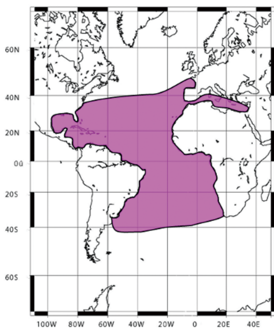
図4. ニシマカジキの分布
