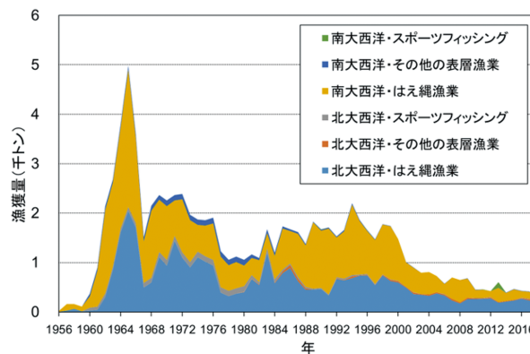
図2. ニシマカジキの海域別・漁法別漁獲量 (ICCAT 2019c)
