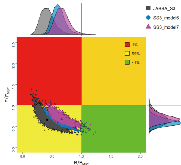
図6. 資源評価結果 (神戸プロット) (ICCAT 2019a)
