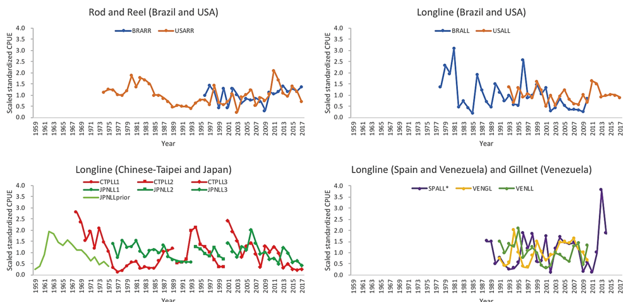
図5. 資源評価で用いられた漁業別資源量指数 (ICCAT 2019a)
