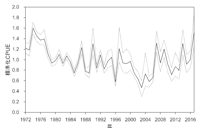
図 8. 太平洋北区における沖底（かけまわし漁法）の標準化 CPUE 標準化 CPUE は 1 が平均値となるように基準化、破線は 95%信頼区間の上限値と下限値。
