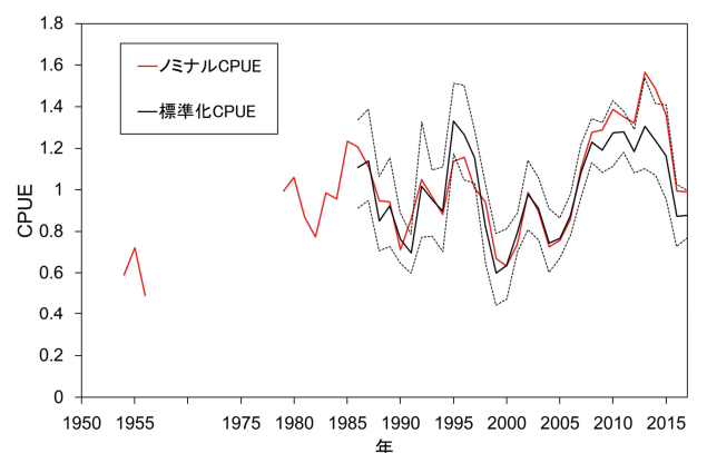
図 9. 津軽海峡内で操業を行う底はえ縄のノミナル CPUE（標準化されていない CPUE）と標準化 CPUE 1986～2012 年の三厩および 2007～2017 年の大間の漁獲データを用いた（各 CPUE は 1 が平均値となるように基準化、破線は 95%信頼区間の上限値と下限値）。1957～1978 年のデータはない。
