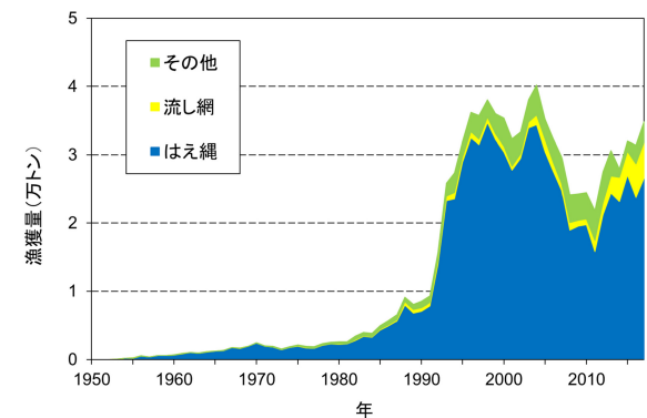
インド洋におけるメカジキの漁法別漁獲量（1950～2017年）（IOTC データベース：2018年12月） 2017年は暫定値。
