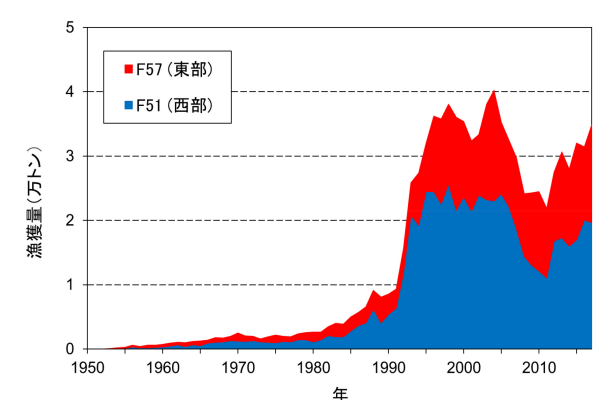
インド洋におけるメカジキのFAO 海域別漁獲量（1950～2017年）（IOTC データベース：2018年12月） 2017年は暫定値。
