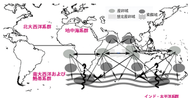
インド洋におけるメカジキの産卵域および索餌域
