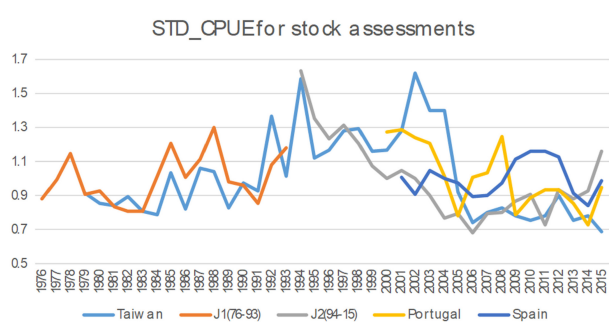
資源評価で使用されたメカジキはえ縄標準化 CPUE J1 は日本はえ縄前期、J2 は後期。
