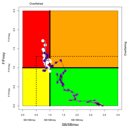
SS3 による資源評価結果（神戸プロット、白丸はベースの 24 通りのグリッド解析による 2017 年の資源状態、灰色の丸はメディアン）
