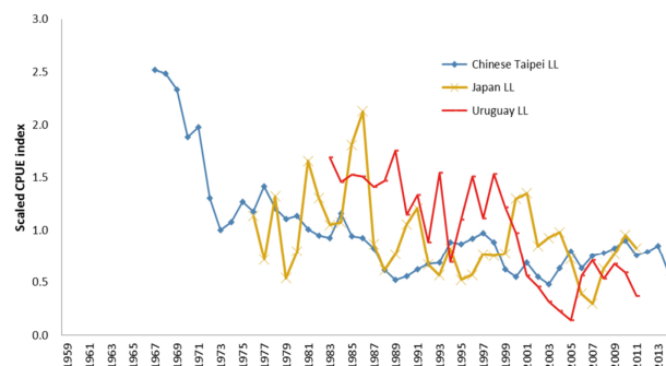
図 5. 2016 年の資源評価に用いられた南大西洋ビンナガの標準化 CPUE (ICCAT 2016)
