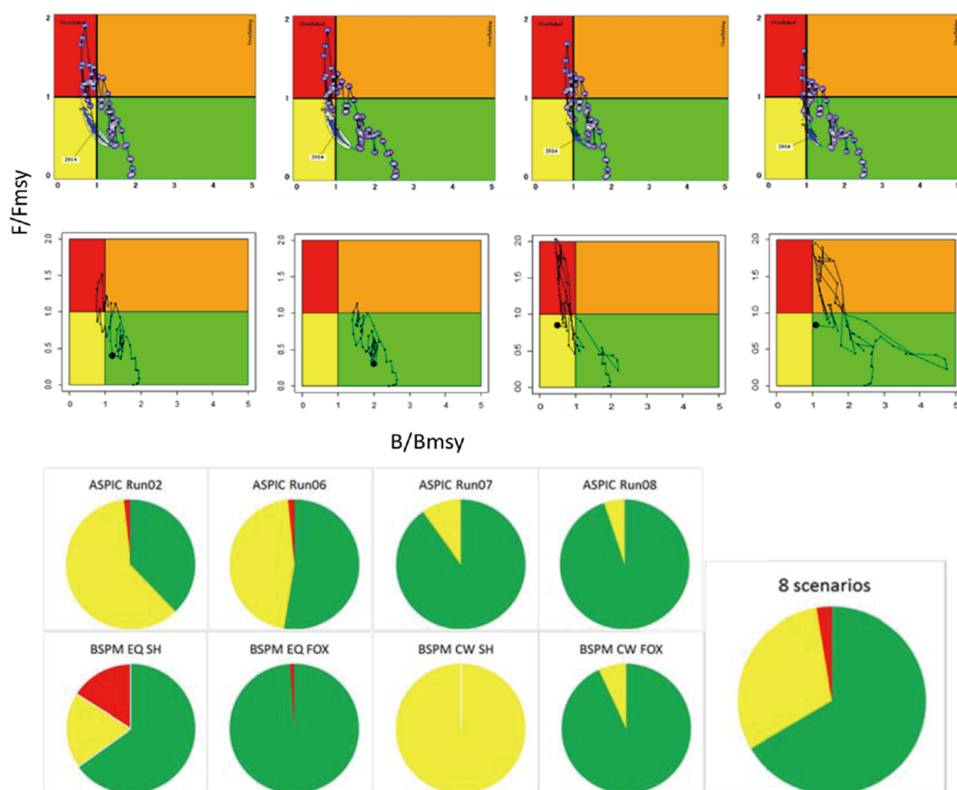
図 4. 資源評価における BSP および ASPIC モデルのそれぞれシナリオごとの Kobe plot (上段) と資源状態を確率として示した円グラフ (下段)
