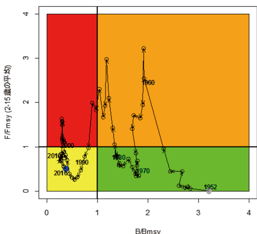
図 4. 神戸プロットの一例。ミナミマグロの資源量と漁獲水準の経年変化を示す（高橋ほか 2018） 右下の領域（緑）では、資源量が B_{MSY} より多く、漁獲水準が F_{MSY} より低い状態である。一方、左上の領域（赤）では、資源量が B_{MSY} より少なく、漁獲水準が F_{MSY} より高い状態である。
