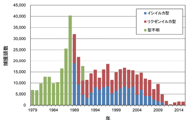
イシイルカ捕獲頭数の推移 (1979～2015年)
