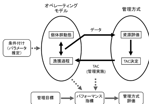
図 5. オペレーティングモデルを利用した管理方式の開発の概念図 (Kurota et al. 2010 を改変)。シミュレーションにより、管理方式の性能が評価され、最適なものを選ばれる。
