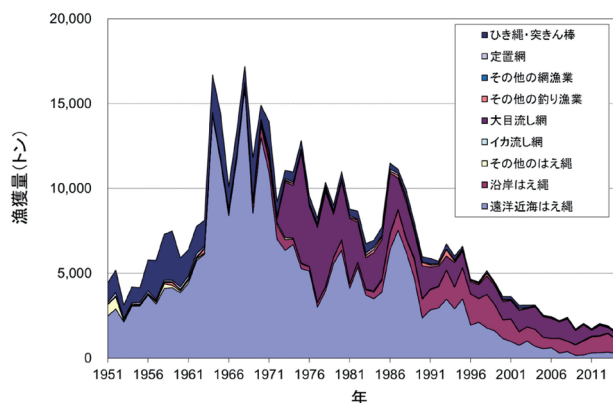
図 1. 北太平洋（赤道以北）におけるマカジキの我が国の漁業種別漁獲量（ISC 2015）
