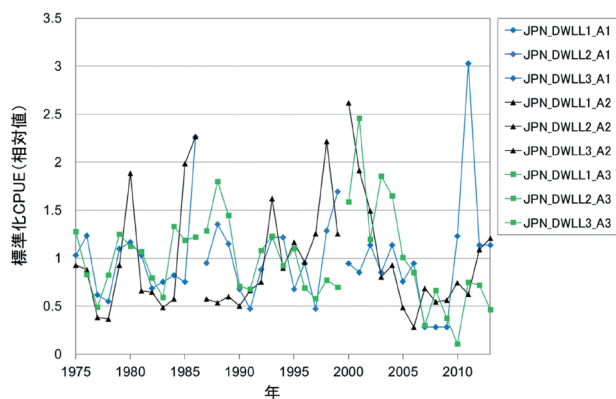
図4. 資源評価に用いた日本の遠洋近海はえ縄の資源量指数 青：エリア 1（北緯 10 度以南）、黒：エリア 2（北緯 10 度以北かつ東経 160 度以西）、緑：エリア 3（北緯 10 度以北かつ東経 160 度以东）
