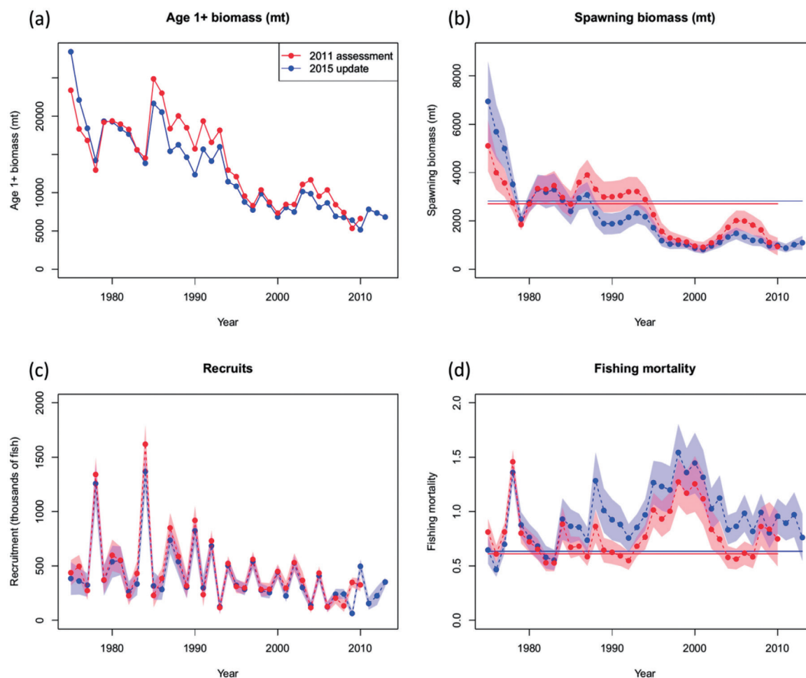
図 6. 統合モデル (Stock Synthesis 3) の解析結果
