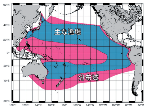
図3. 太平洋におけるマカジキの分布域（桃色）と主要漁獲域（青色） 現在マカジキを主対象とした漁業はごく小規模な沿岸漁業に限られている。マカジキは、主にはえ縄によって漁獲される。
