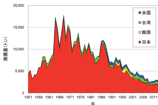
図 2. 北太平洋におけるマカジキの国別漁獲量（ISC 集計分）（ISC 2015）
