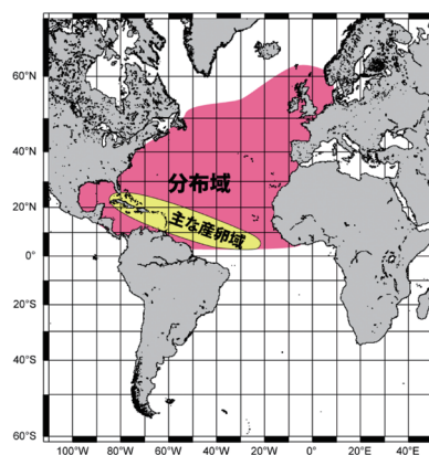
図 4. 大西洋におけるメカジキの分布
