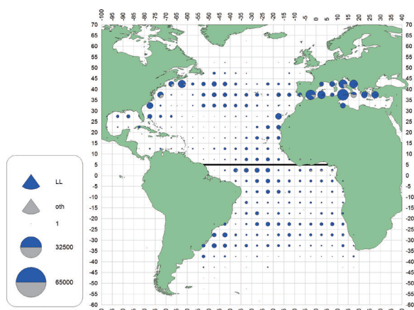
図 3. 大西洋における漁法ごとのメカジキの累積漁獲量（2010～2013 年の合計）の分布図 (ICCAT 2015)
