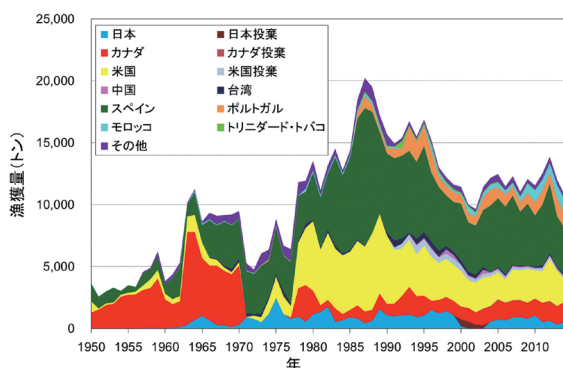
図 1. 北大西洋におけるメカジキの国別漁獲量 (ICCAT 2015) 2014 年の値は暫定値。
