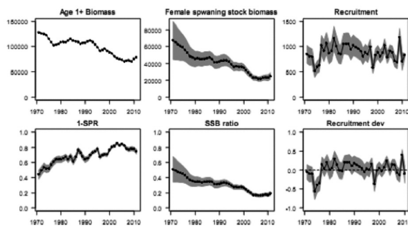
図 5. Stock Synthesis 3 によるベースケースの結果 上図: 左は 1 歳魚以上の資源量、中は雌の産卵親魚量、右は加入量 (×1,000 尾) を示す。下図: 左は加入した雌が産卵群に加入するまでに漁獲される割合、中は処女資源に対する産卵親魚の割合、右は加入量の偏差を示す。実線部分は推定値を、灰色部分は 95% 信頼限界を示す。
