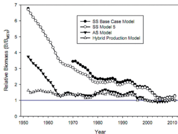
図 6. 異なる資源解析モデルによる資源解析結果 黒丸は Stock Synthesis 3 によるベースケース、白丸はベースケースに 1970 年以前の漁獲量を追加したモデル、白△は Bayesian Surplus Production Model、黒▼は最尤法を用いた Age Structured Model による解析結果を示している。
