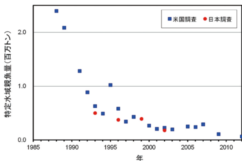
図4. 特定水域における日米調査船調査による中層性スケトウダラの現存量 (親魚量) 推定値 (単位: 百万トン)
