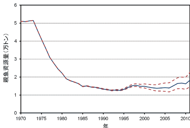
図 4. 大西洋クロマグロ (西系群) の親魚資源重量の経年変化 (ICCAT 2012) 上下の点線間は 80% 信頼範囲。
