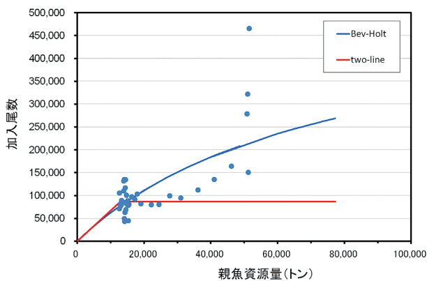
図 6. 大西洋クロマグロ（西系群）の親仔関係（ICCAT 2012） 赤と青線は、将来予測に用いた 2 つの仮定を示す。
