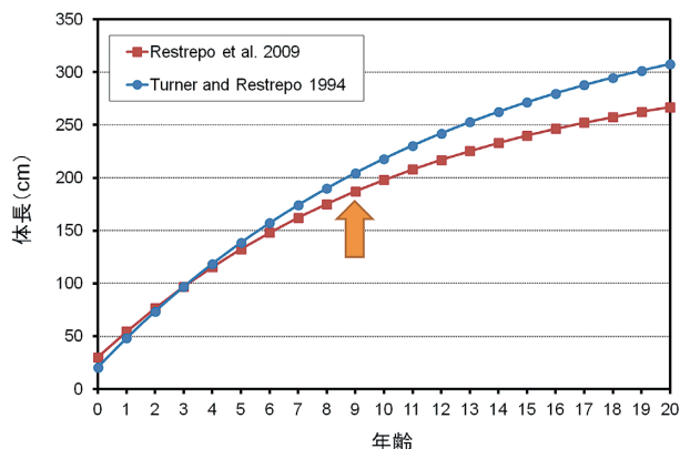
図 3. 大西洋クロマグロ (西系群) の成長曲線 (ICCAT 2011a) 赤は 2010 年の資源評価で更新された成長曲線、青は更新前を示す。図中の矢印は成熟体長を表す。
