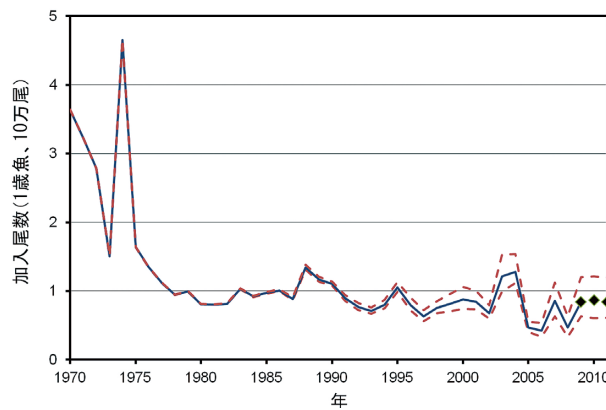
図 5. 大西洋クロマグロ (西系群) の加入量 (1 歳の尾数) の経年変化 (ICCAT 2012) 上下の点線間は 80% 信頼範囲。最近年 (2009 ~ 2011 年) は信頼性が低いためマークを変えた。
