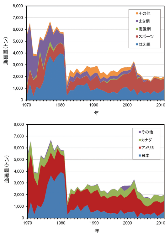
図 2. 大西洋クロマグロ (西系群) の年別漁法別漁獲量 (上) と年別国別漁獲量 (下) (ICCAT 2012) 漁獲量には投棄分も含まれる。
