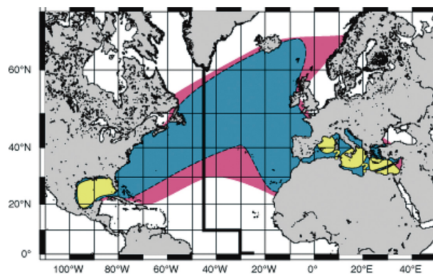
図 1. 大西洋クロマグロの分布域 (赤) と主要漁場 (青)、産卵場 (黄) 索餌場は産卵場を除く海域。縦太線は東西の系群の区分。
