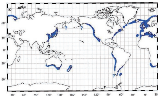
ウバザメの分布 (Last and Stevens, 1994)
