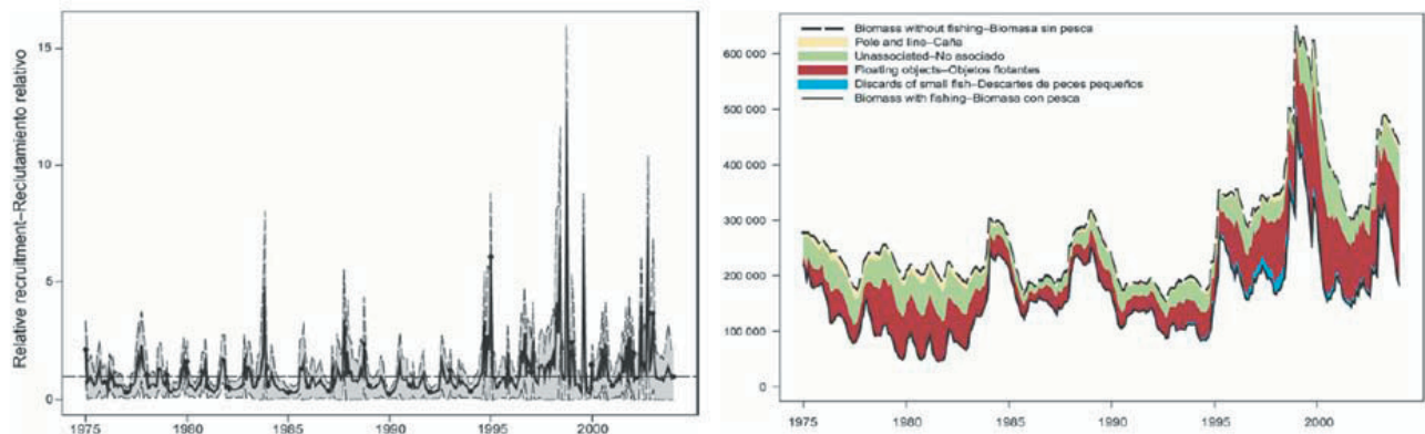
図5. A-SCALAで推定したカツオの加入量(平均に対する相対値、左)と資源量(千トン、右)(Anon 2006)
