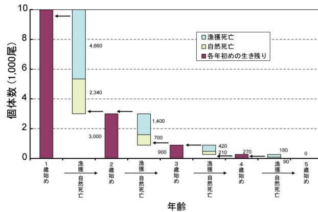
図 6. VPA による資源尾数の推定の基本原理。
