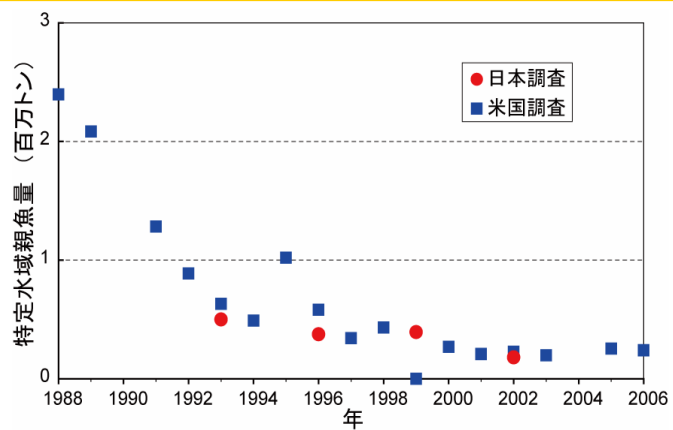
条約特定水域における日米調査船調査による中層性スケトウダラの現存量(親魚量)推定値
