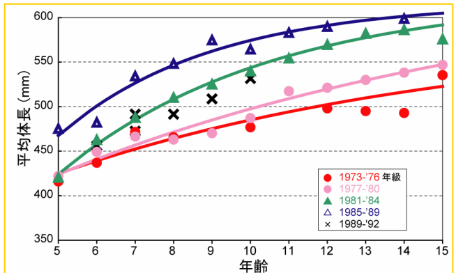
アリューシャン海盆のスケトウダラ(雌)年齢と体長の関係
