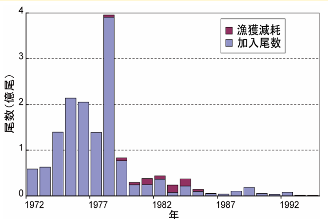
条約特定水域で米国調査により捕捉された7歳魚加入尾数(1988年以前の加入尾数は生残率から逆算された推定値を使用)
